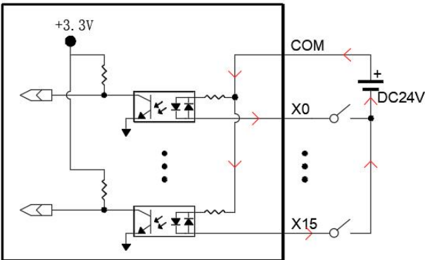
图 2- 5 DI 湿接点 NPN 接线方式
