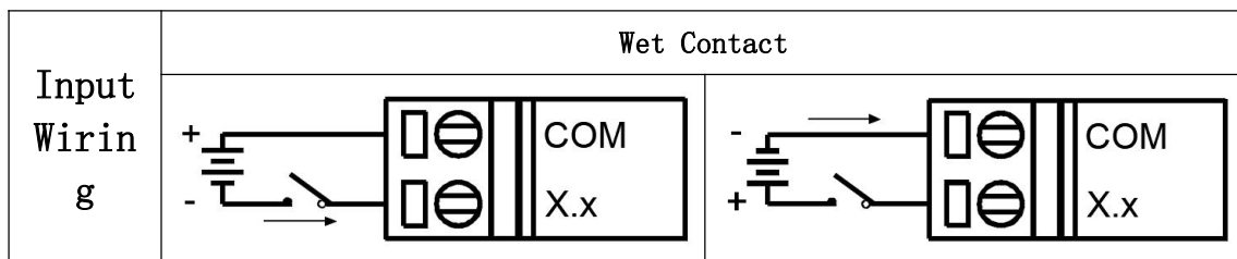
图 4- 1 DI 电气接线图
