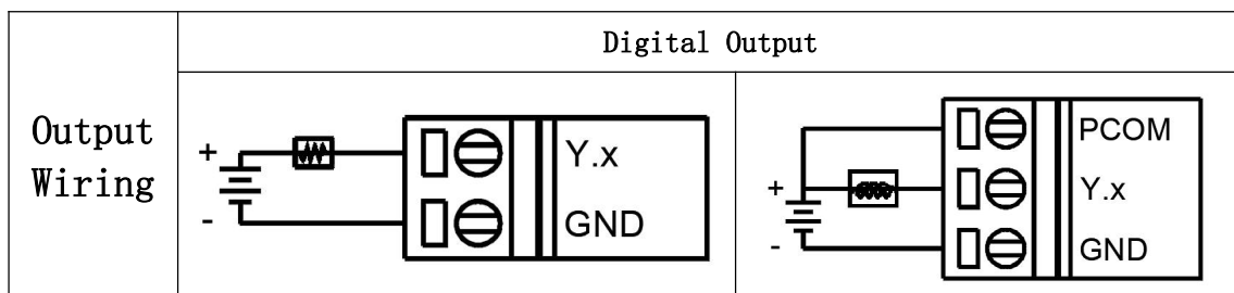
图 4- 2 DO 电气接线图
