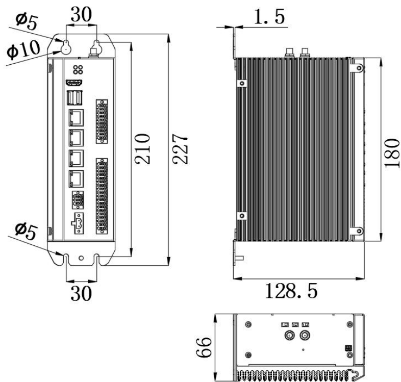
图 2- 1 安装尺寸图
